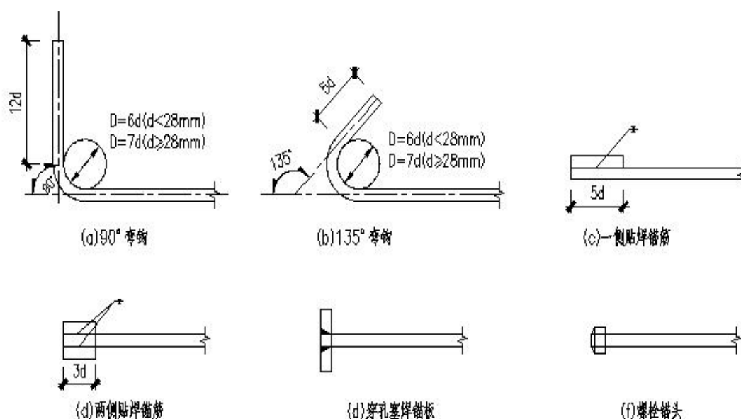
图 6.2.3 弯钩和机械锚固的形式和技术要求
