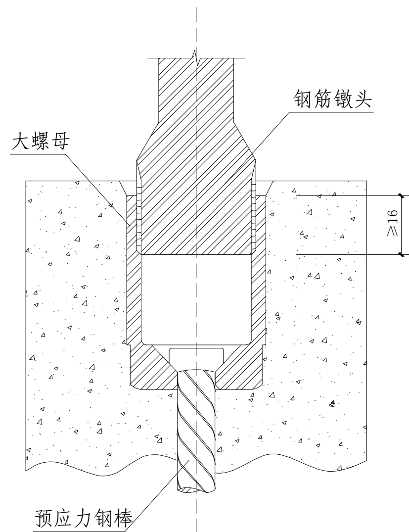
钢筋墩头与大螺帽连接图
