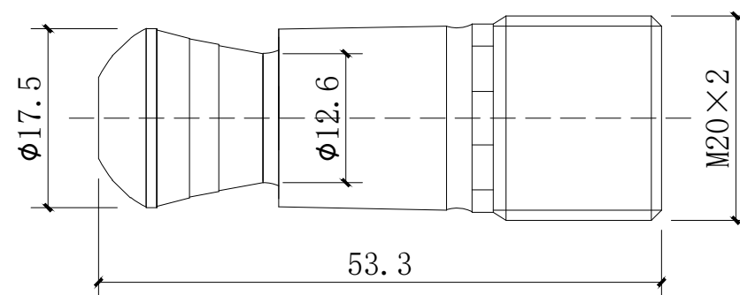
插杆
