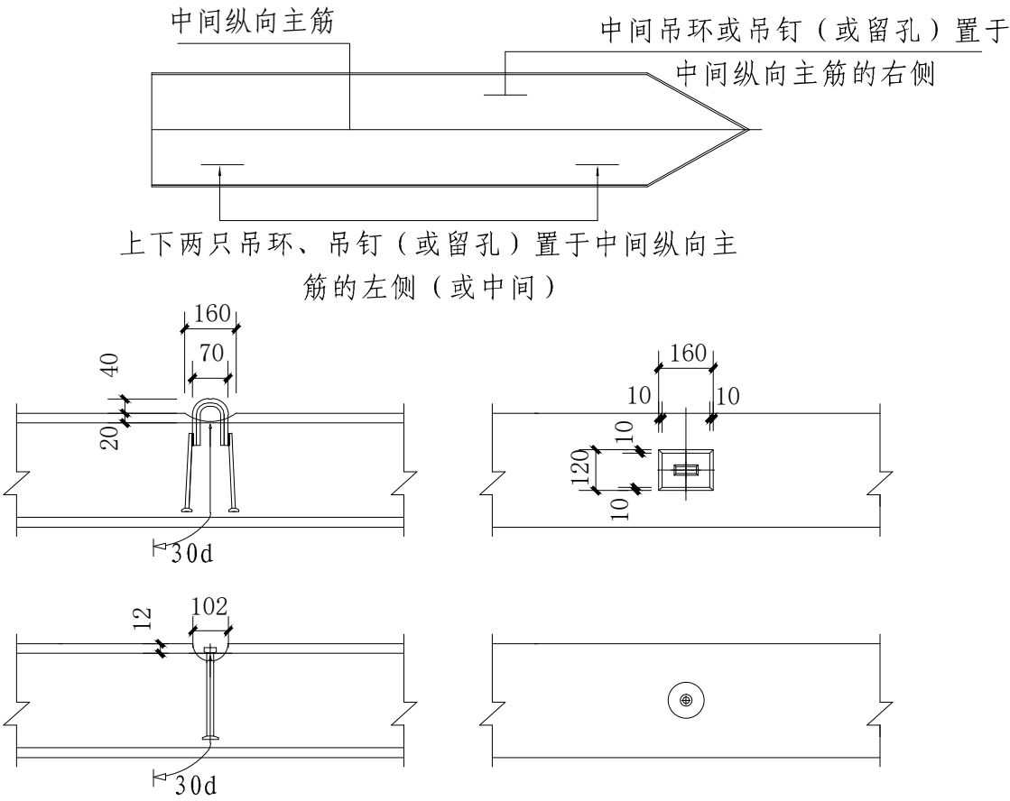
图9.6 方桩预埋吊环或吊钉大样图
