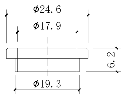
垫圈
