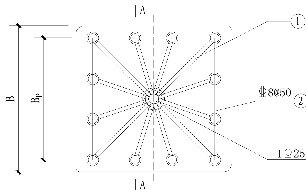
b型桩尖平面图
