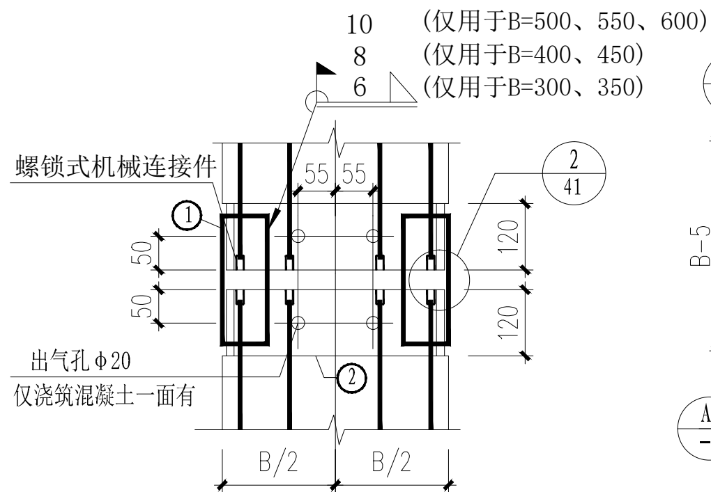
上下节桩连接尺寸示意
