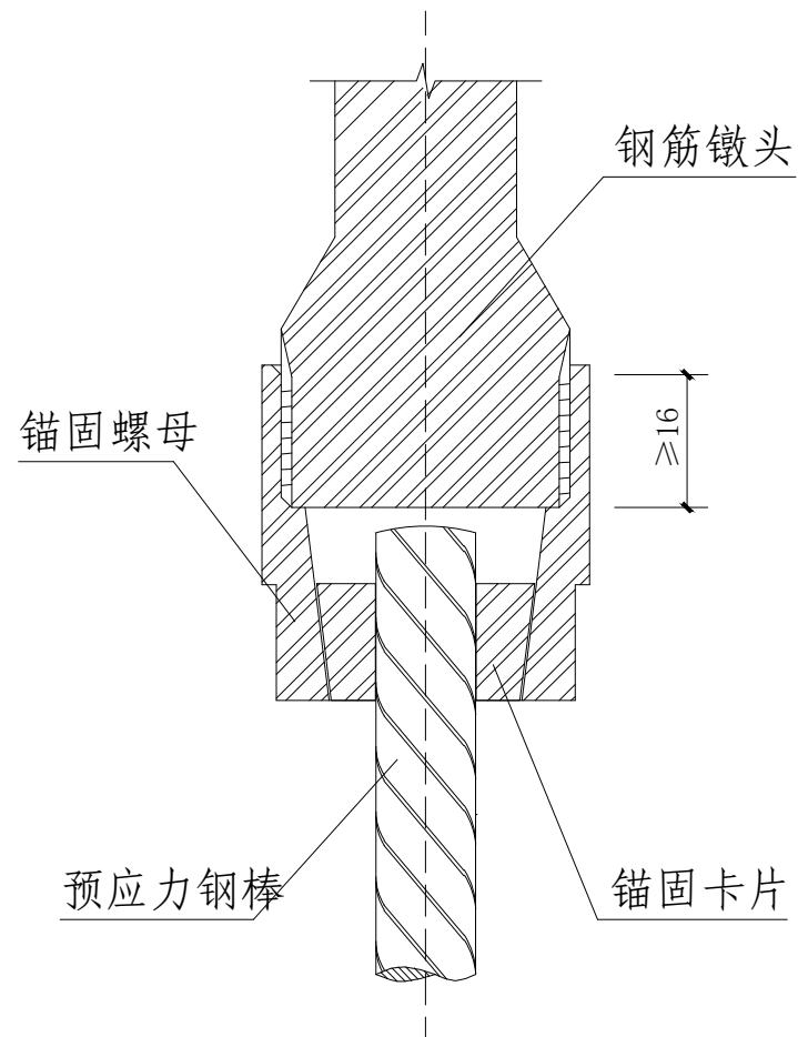
锚固卡片剖面图
