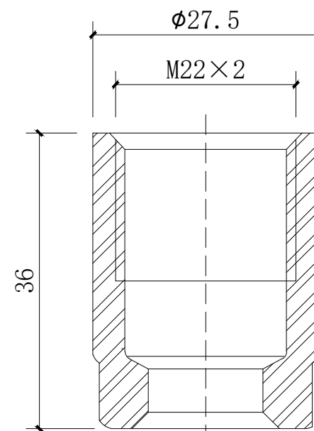
B-B
