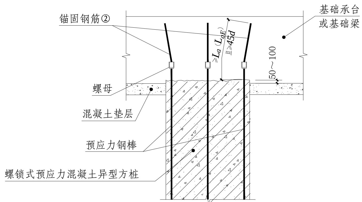
② 抗拔桩截桩桩顶与承台连接详图
