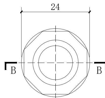
小螺母
