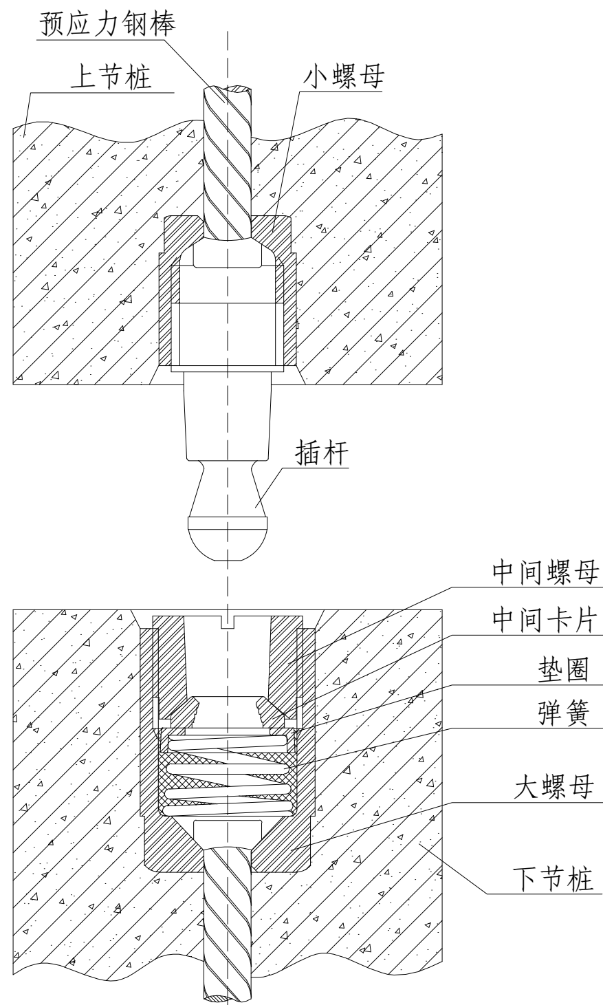
接桩对孔位图
