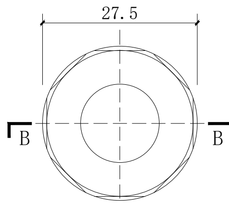
小螺母
