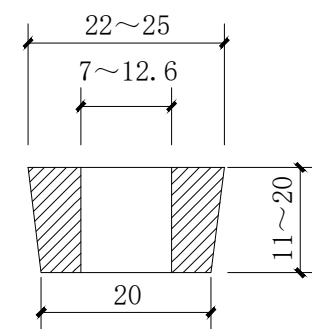
锚固卡片剖面图
