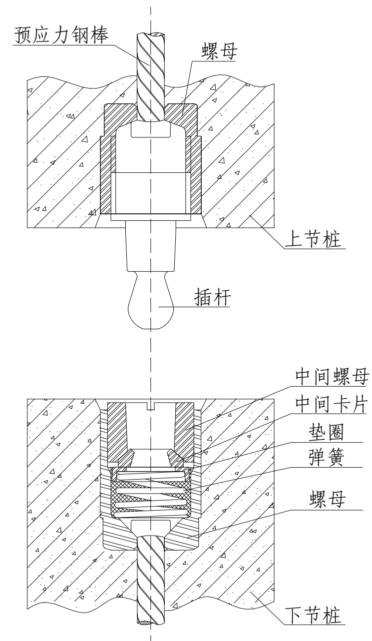
接桩对孔位图
