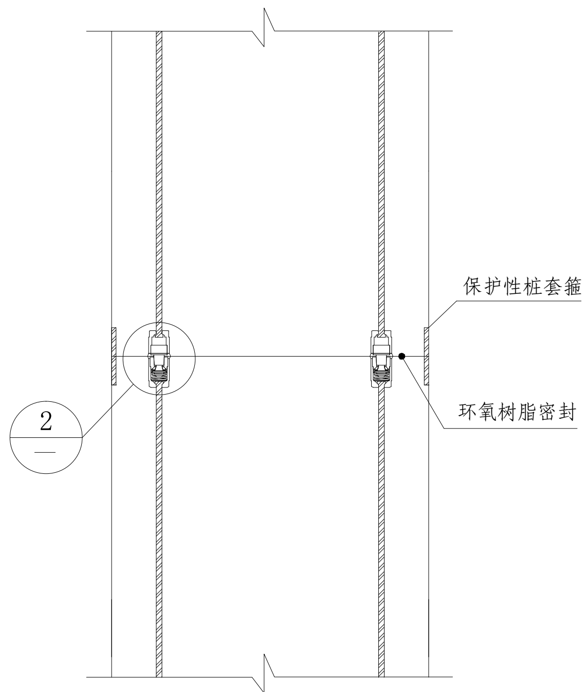
① 机械连接详图
