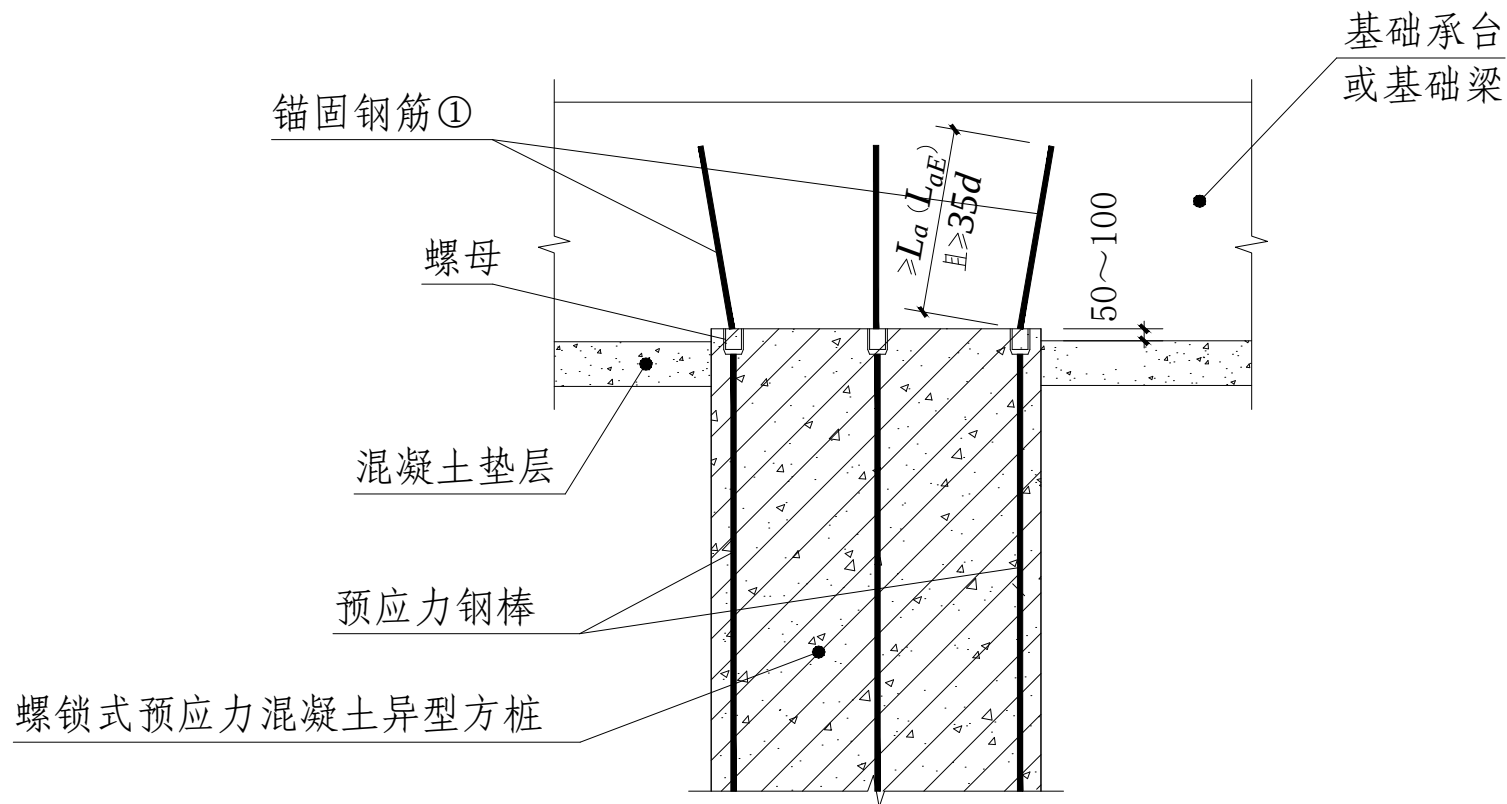
① 抗压桩不截桩桩顶与承台连接详图
