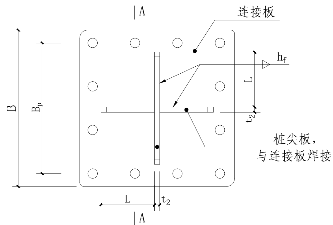
a型桩尖平面图
