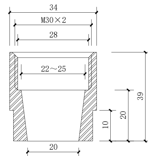
锚固螺母大样图
