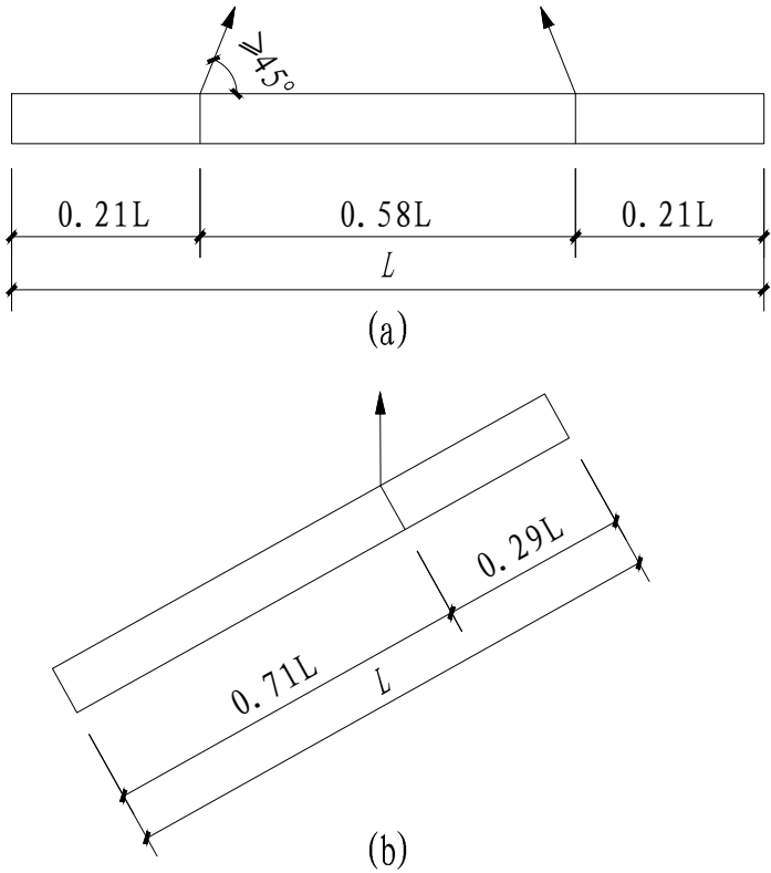
图9.5 方桩起吊方式
