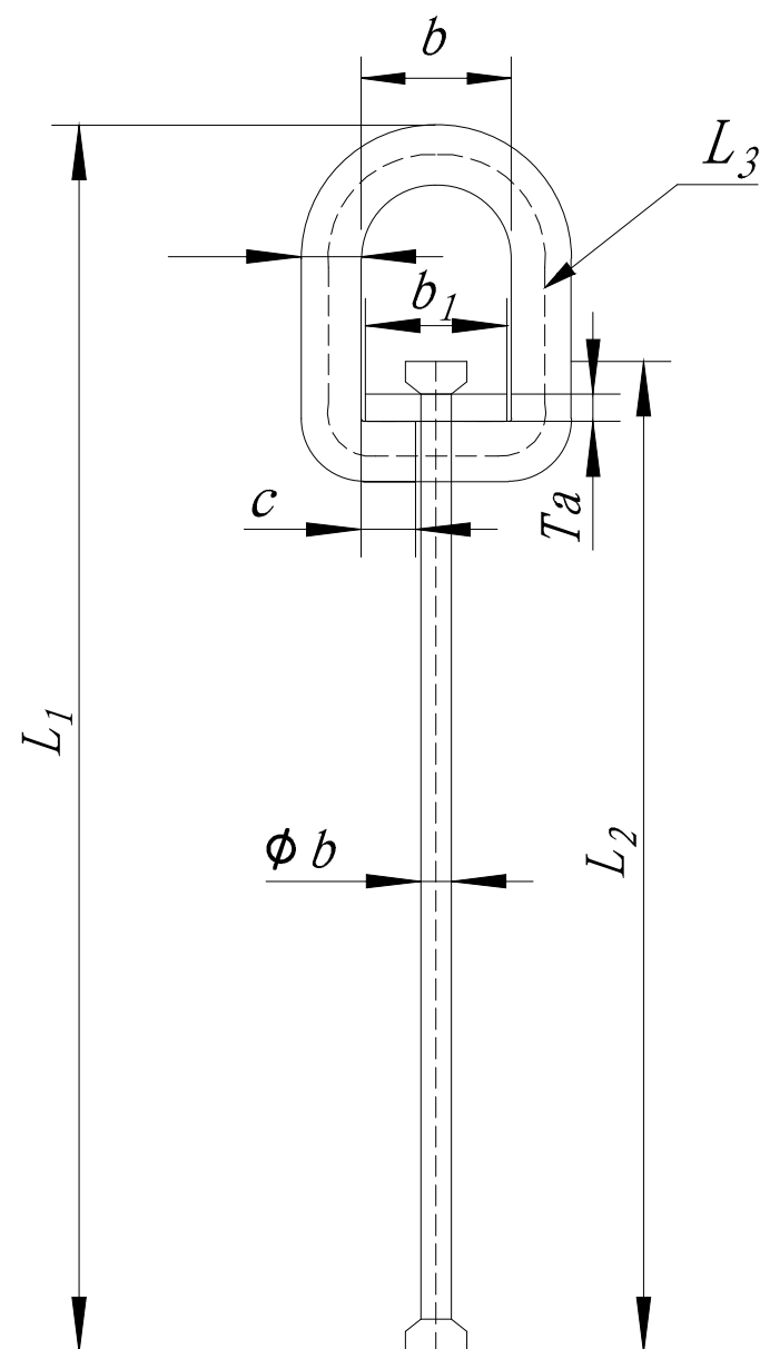
吊环构造大样图 (A型)
