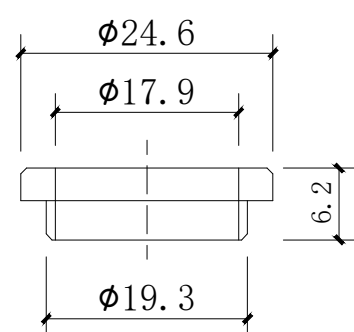
垫圈
