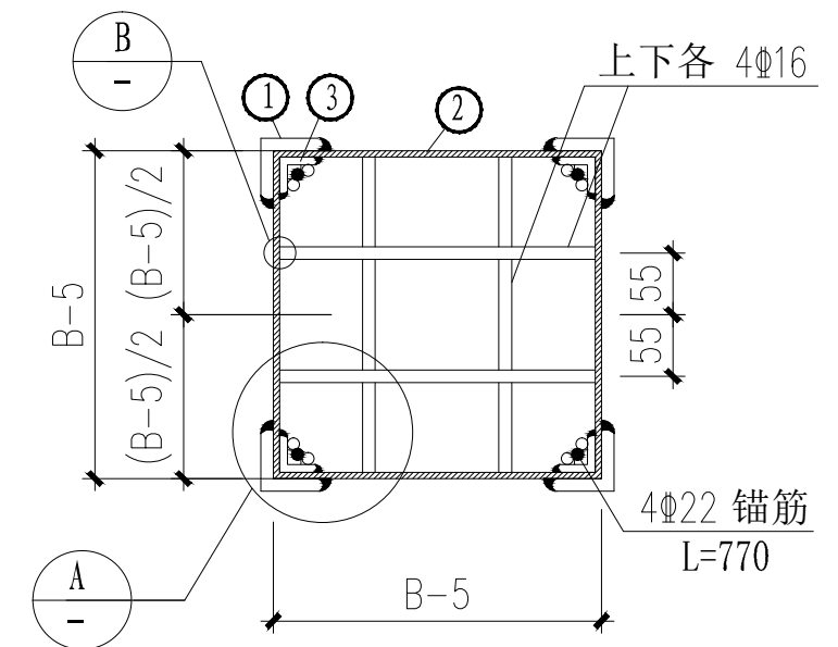
连接平面图
