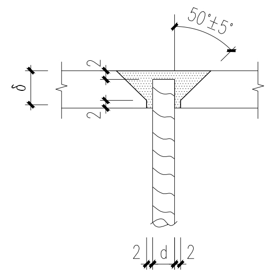
穿孔塞焊详图
