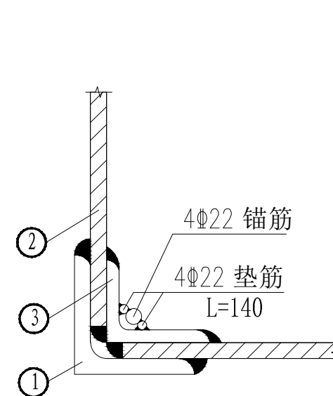
上下节桩连接尺寸示意
